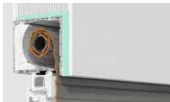
Außen verputzbar KARO + RA.2 (Abb. RA.2)
